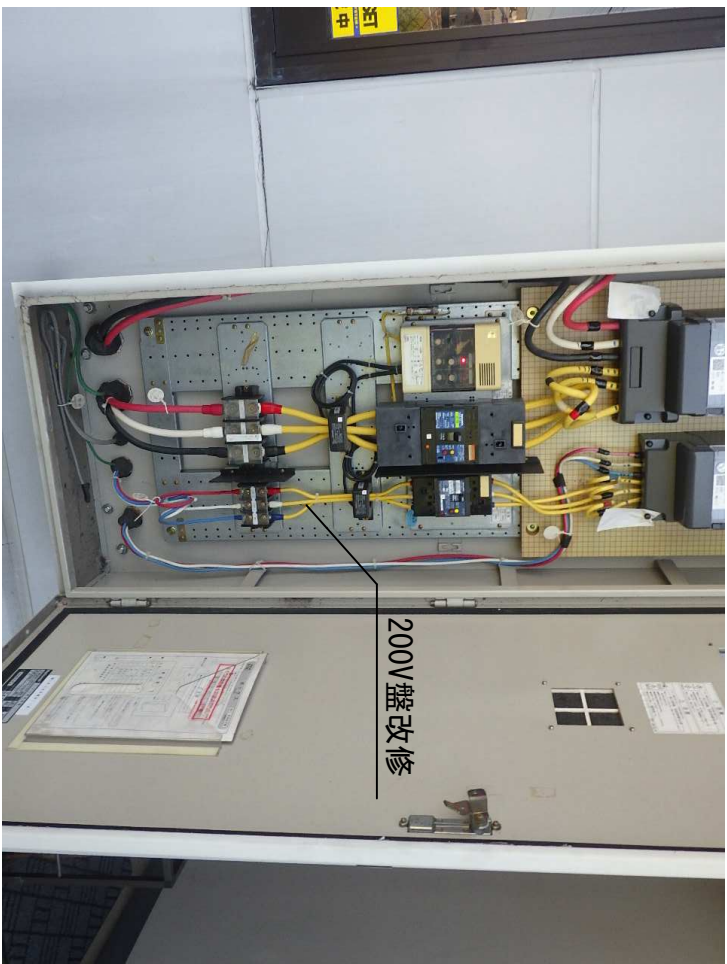
動力盤
